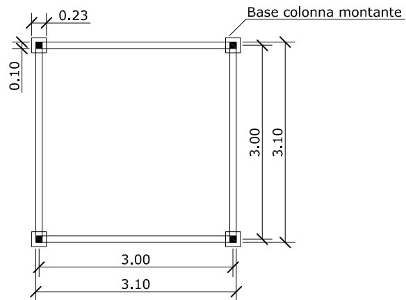
- PIANTA
