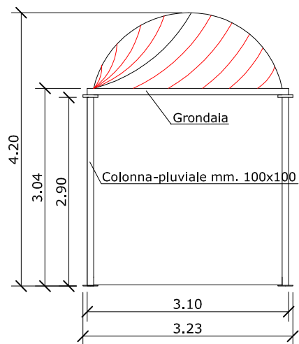
- PROSPETTO
